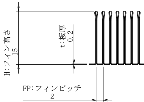
詳細図 A スケール 8 : 5
