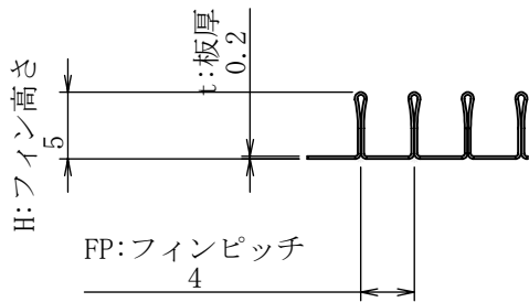
詳細図 A スケール 8 : 5
