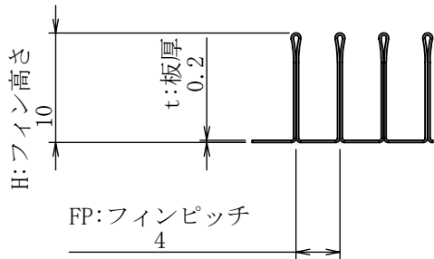
詳細図 A スケール 8 : 5
