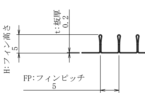
詳細図 A スケール 8 : 5
