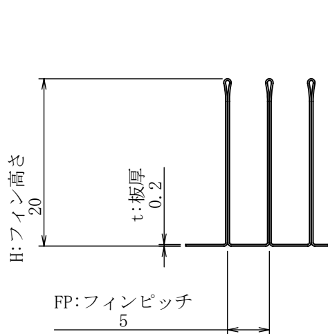
詳細図 A スケール 8 : 5
