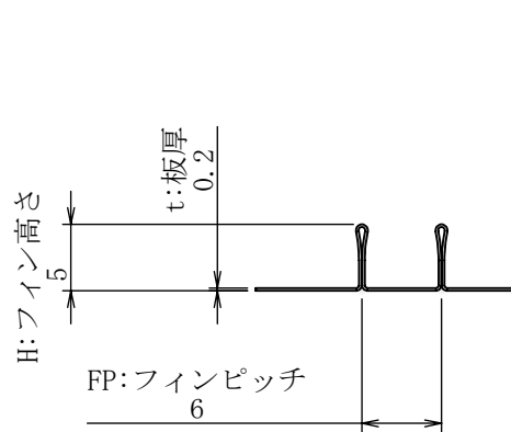
詳細図 A スケール 8 : 5
