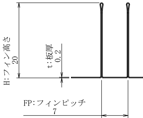
詳細図 A スケール 8 : 5
