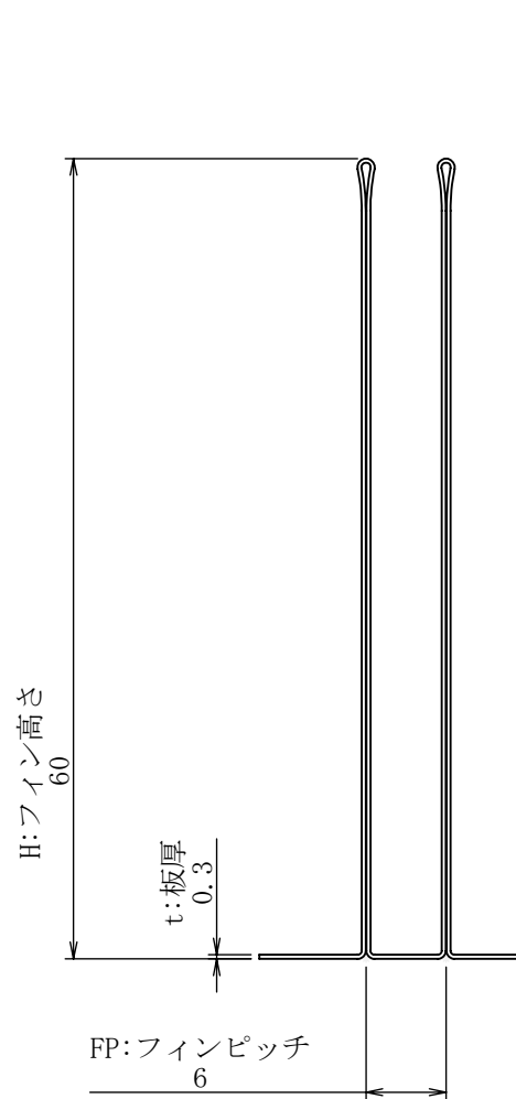
詳細図 A スケール 8 : 5
