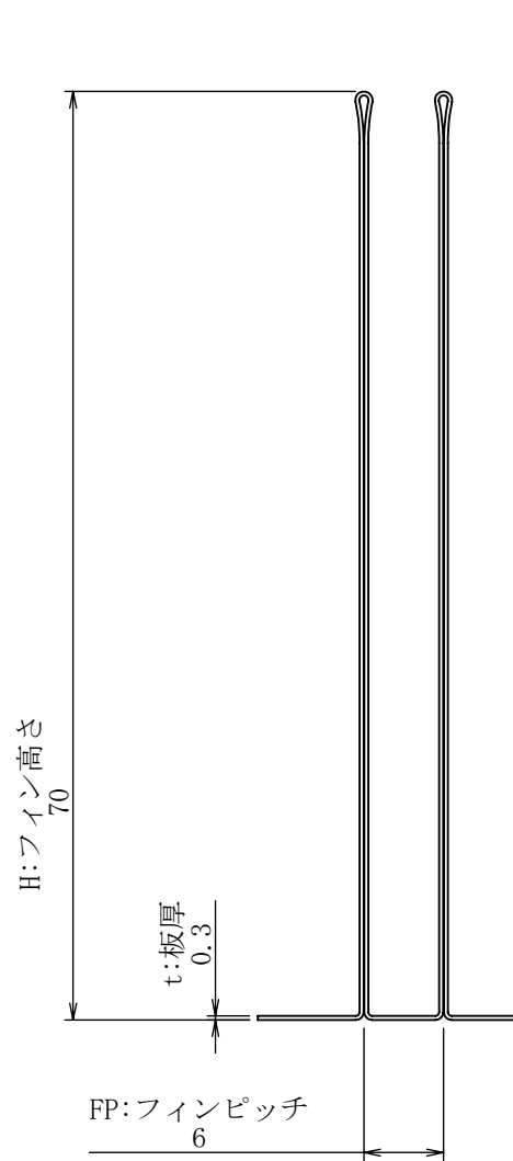
詳細図 A スケール 8 : 5
