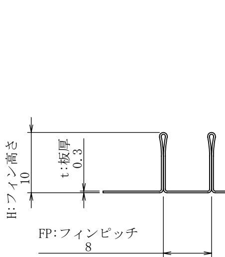
詳細図 A スケール 8 : 5
