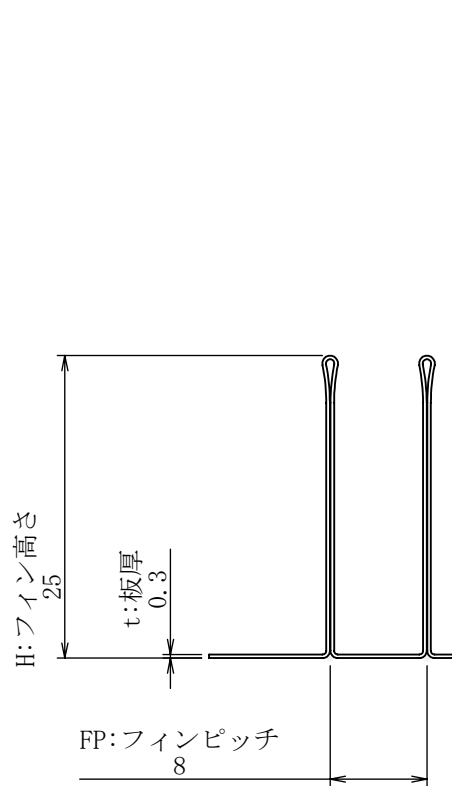
詳細図 A スケール 8 : 5
