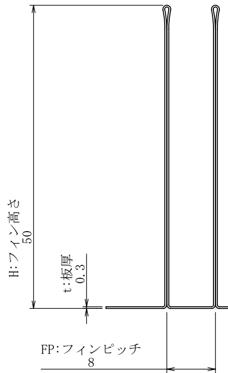
詳細図 A スケール 8 : 5
