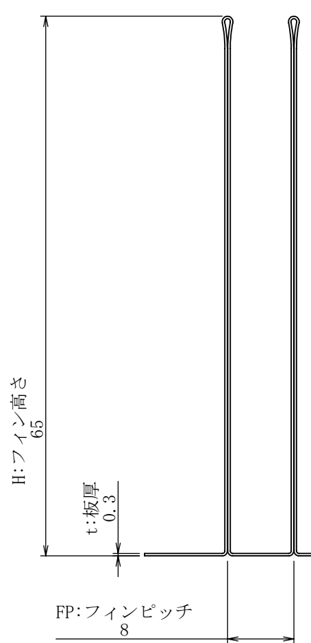
詳細図 A スケール 8 : 5
