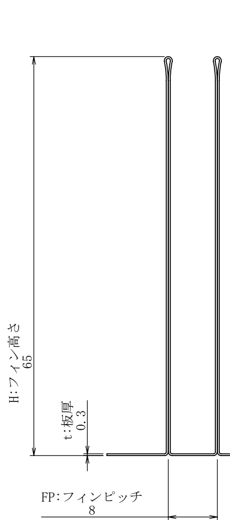
詳細図 A スケール 8 : 5
