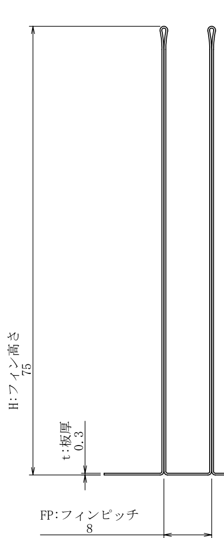
詳細図 A スケール 8 : 5
