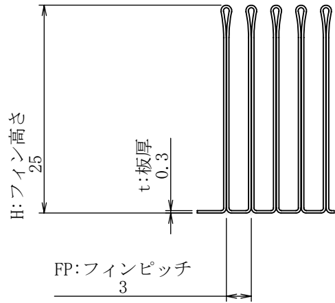
詳細図 A スケール 8 : 5
