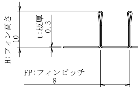
詳細図 A スケール 8 : 5
