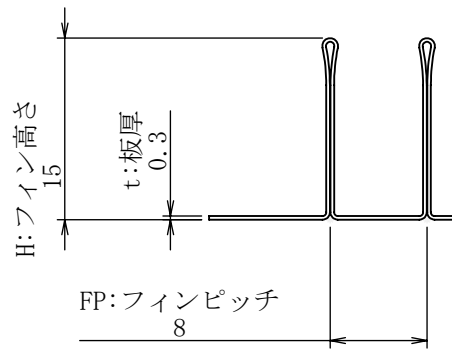
詳細図 A スケール 8 : 5
