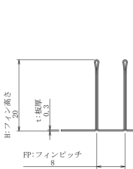
詳細図 A スケール 8 : 5
