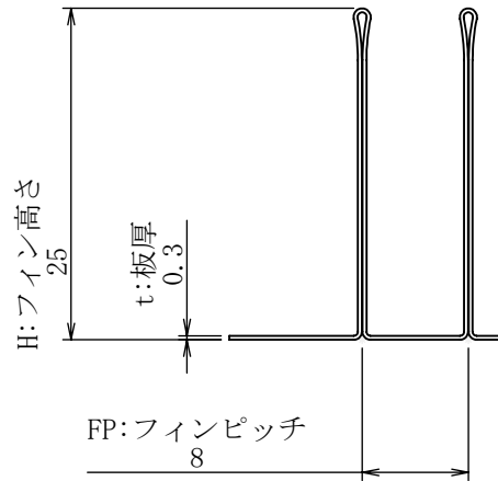
詳細図 A スケール 8 : 5
