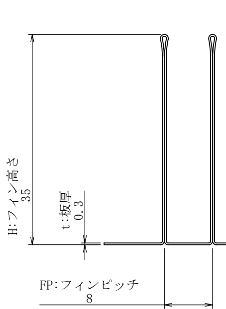
詳細図 A スケール 8 : 5
