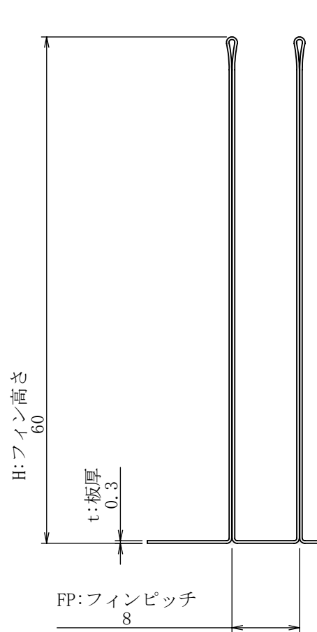
詳細図 A スケール 8 : 5
