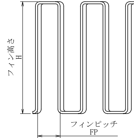
詳細図 A スケール 5 : 1
