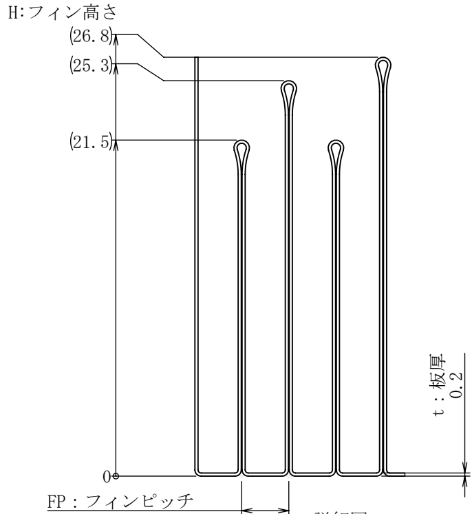
詳細図 A スケール 3 : 1
