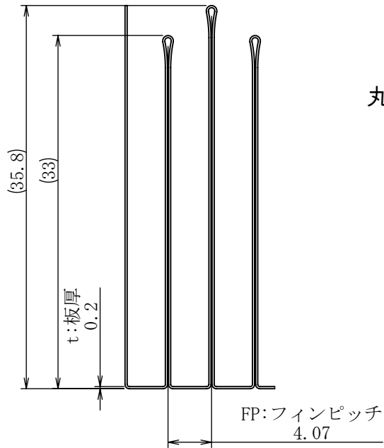
詳細図 A スケール 2 : 1
