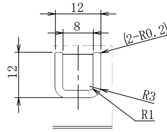
詳細図 C スケール 1 : 1
