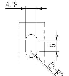
詳細図 D スケール 1 : 1
